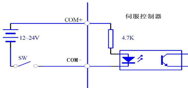
图 4.6 开关量输入接口
