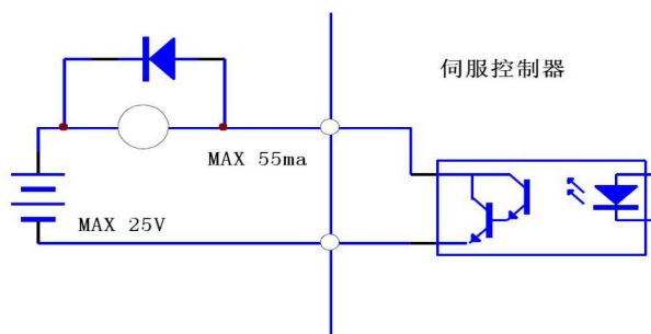
图 4.7 开关量输出接口
