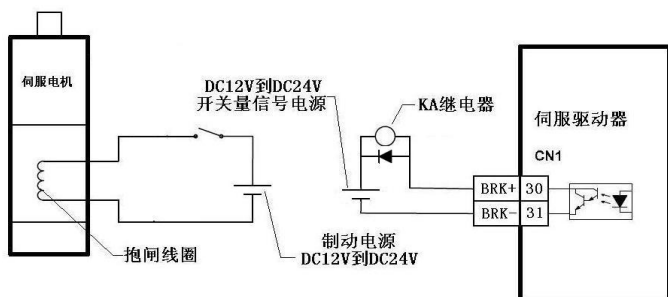
图 3.5 抱闸电机接线图
