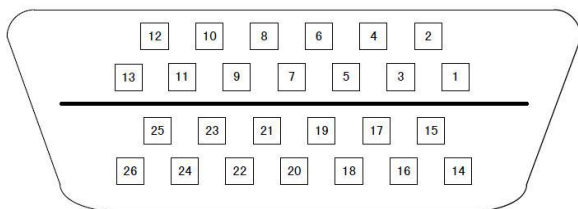
图 4.3. 面对 CN2 26 芯插头焊片
