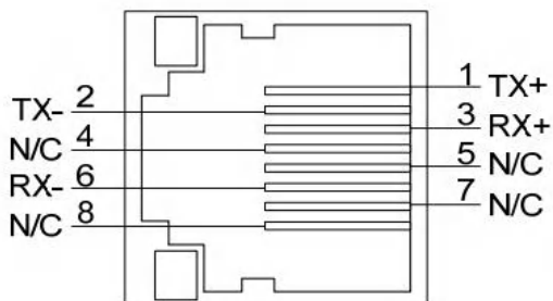
图 4.5 面对 CN6/CN7 插头焊片看
