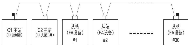
MechatrolinkII/III连接形式
