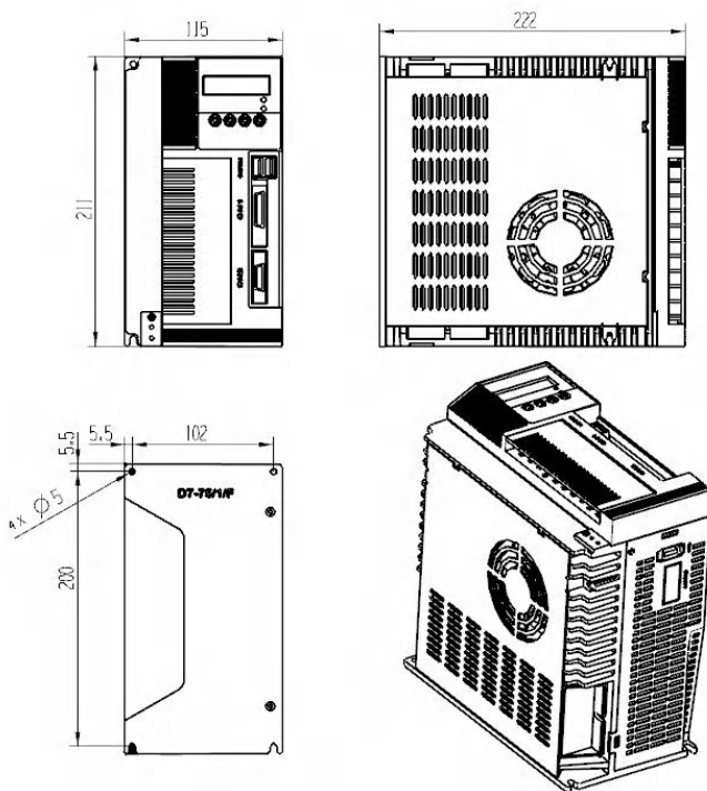
图1.1.4 25A/50A/75A 外观尺寸图
