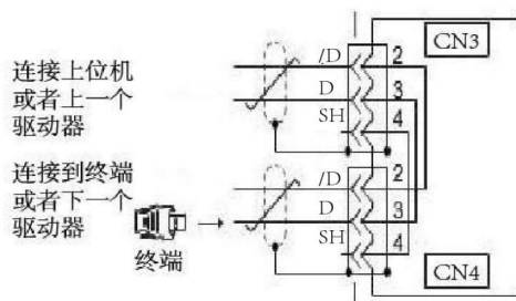
图 3.4.3 总线连接图
