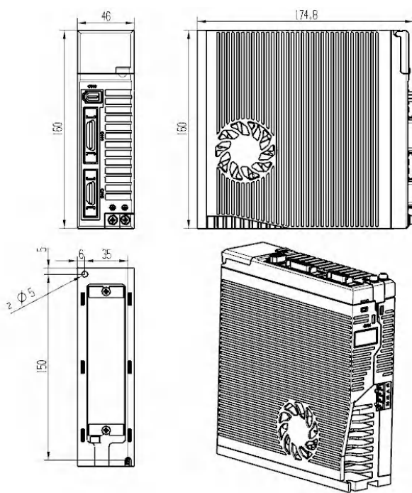
图1.1.1 10A/22A/32A 外观尺寸图
