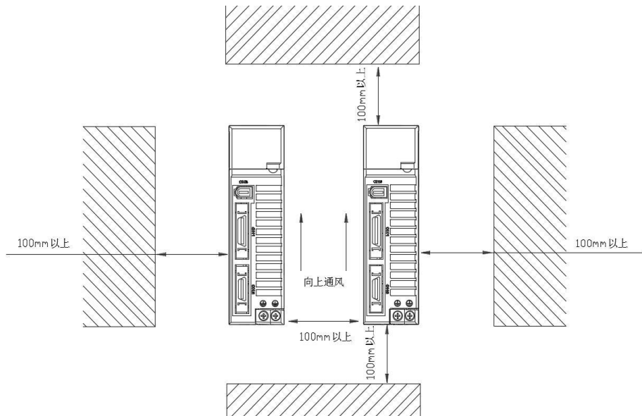
图1.4 安装方位
