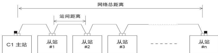
MechatrolinkII 的连接形式(不使用中继器时)
