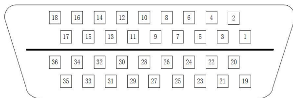
图 4.2 面对 CN1 36 芯插头焊片看
